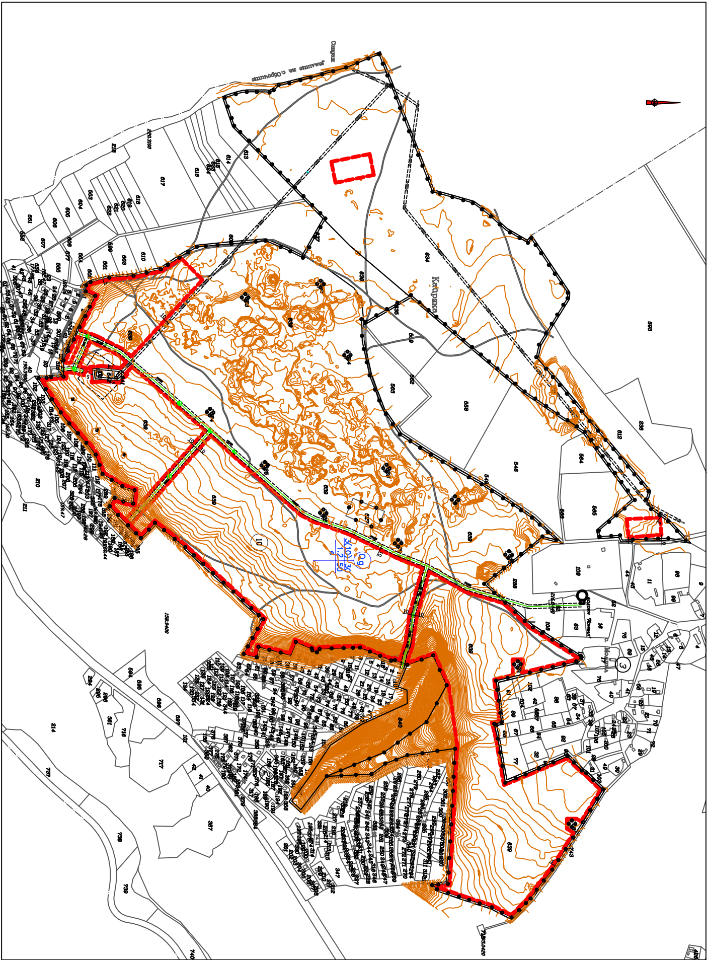
ПЛАН ЗА ЗАСТРОВАВАНЕ за ПИ 02508.10.634, ПИ 02508.10.636, ПИ 02508.10.639 на в.з. "Мончили" на гр.България, отредени за "Ваканционно селище Мончи-гоф и Голф-трипе " " М 1 : 10000
