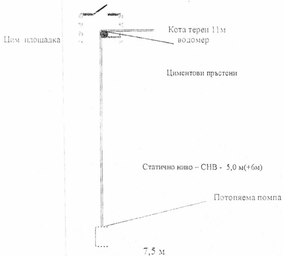
Фиг.1. Конструкция на ШК "Извора-Кранево"
